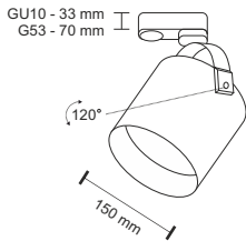
Lampa wykonana ze stali, aluminium i tworzywa sztucznego. System bezśrubowy. Nie zawiera źródła światła. / The lamp is made of steel, aluminium and plastic. No screw connections. Light source not included.
