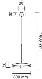
Lampa wykonana ze stali i aluminium. System bezśrubowy. Wbudowane źródło światła. / The lamp is made of steel and aluminium. No screw connections. Light source included.
