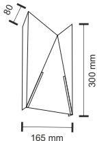
Lampa wykonana ze stali i aluminium. System bezśrubowy. Nie zawiera źródła światła. / The lamp is made of steel and aluminium. No screw connections. Light source not included.
