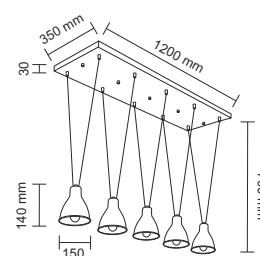
Lampa wykonana ze stali i aluminium. System bezśrubowy. Nie zawiera źródła światła. / The lamp is made of steel and aluminium. No screw connections. Light source not included.
