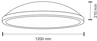
Lampa wykonana ze stali, aluminium i plexi. Obudowa laminat poliestrowo-szkłany. System bezśrubowy. Nie zawiera źródła światła. / The lamp is made of steel, aluminium and plexiglas. The housing is made of polyester-glass laminate. No screw connections. Light source not included.
