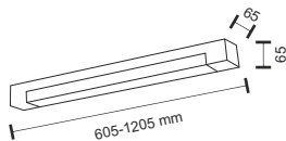
Lampa wykonana ze stali i aluminium. System bezśrubowy. Wbudowane źródło światła. / The lamp is made of steel and aluminium. No screw connections. Light source included.
